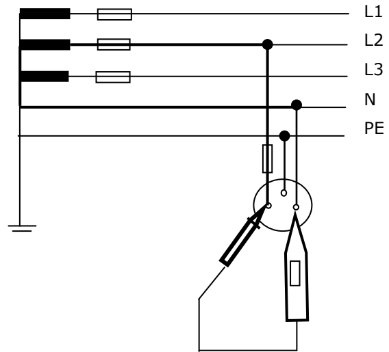
Obr: Meranie vnútorného odporu siete
