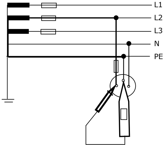
Obr: Meranie impedancie ochrannej slučky
